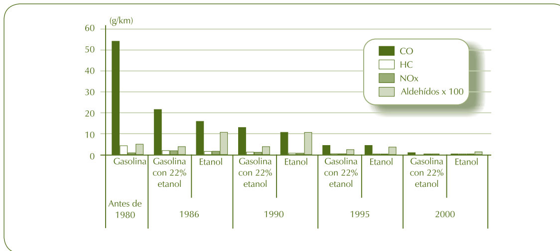
Gráfico 4 – Evolución de las emisiones de vehículos nuevos en Brasil
