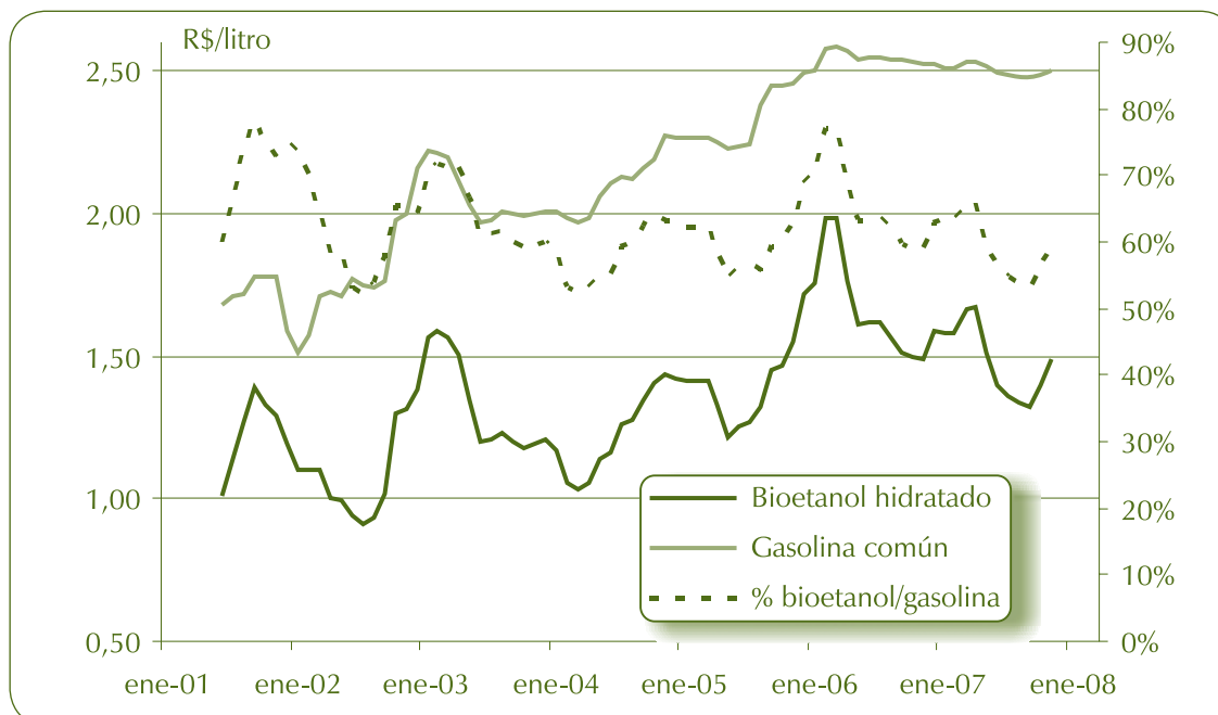
Gráfico 32 – Evolución de los precios promedio pagados por el consumidor de bioetanol hidratado y de gasolina común y análisis de la relación entre estos precios en Brasil
