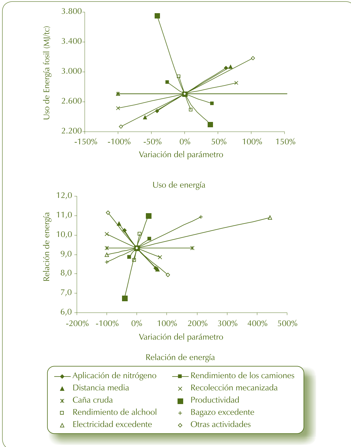
Figura 16 – Análisis de sensibilidad del uso de la energía y de relación consumo/ producción de energía en la producción de caña de azúcar en el escenario actual (2005/2006)
