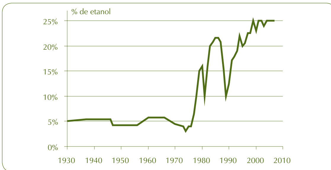
Gráfico 17 – Promedio de concentración de etanol anhidro en la gasolina brasileña
