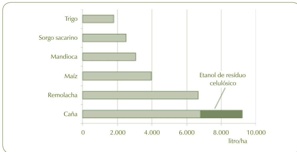
Gráfico 8 – Productividad promedio de etanol por área para diferentes cultivos energéticos
