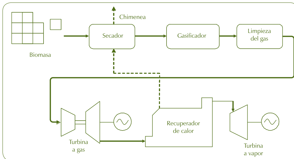
Figura 20 – Representación esquemática de un sistema BIG/GT-CC
