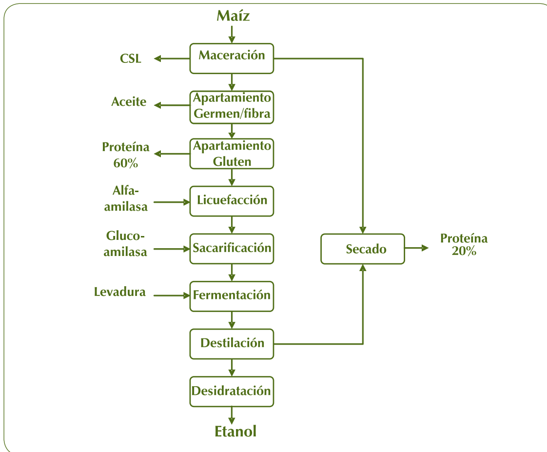
Figura 13 – Organigrama del proceso de molienda húmeda para la producción de bioetanol con maíz
