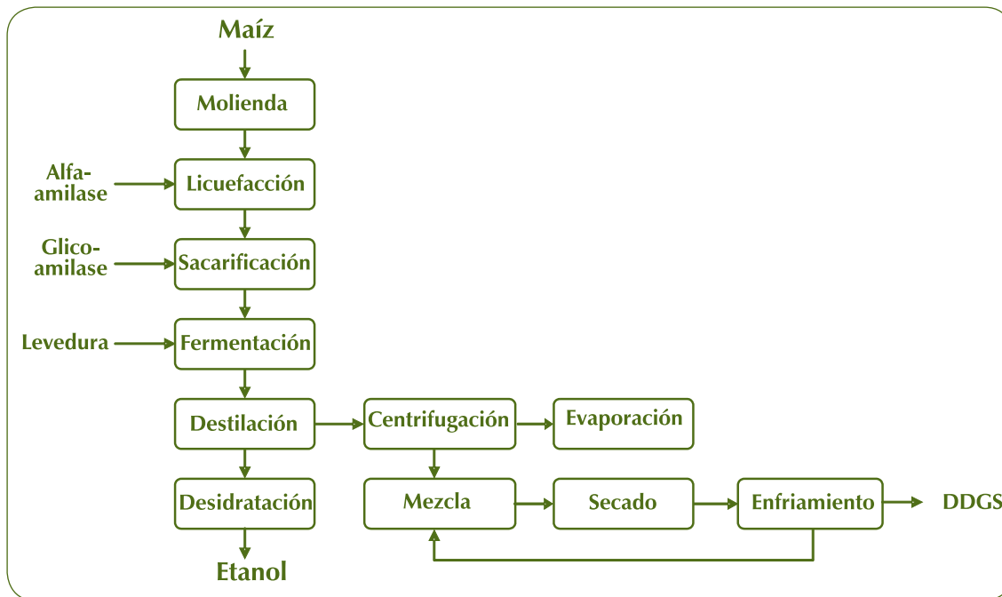
Figura 14 – Organigrama del proceso de molienda seca para la producción de bioetanol con maíz
