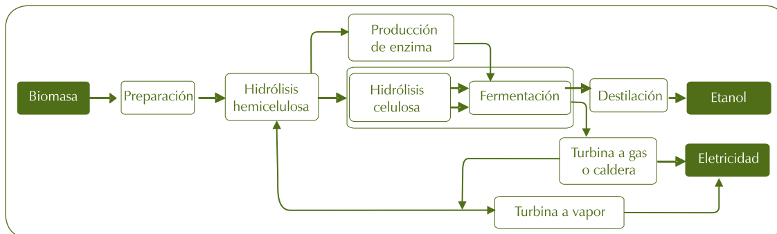
Figura 19 – Esquema del proceso de producción de etanol por medio de la hidrólisis de la biomasa
