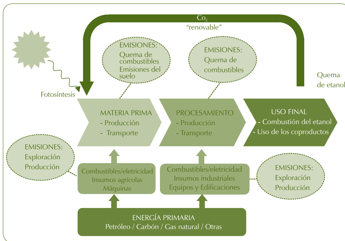
Figura 15 – Diagrama del ciclo de vida de un biocombustible
