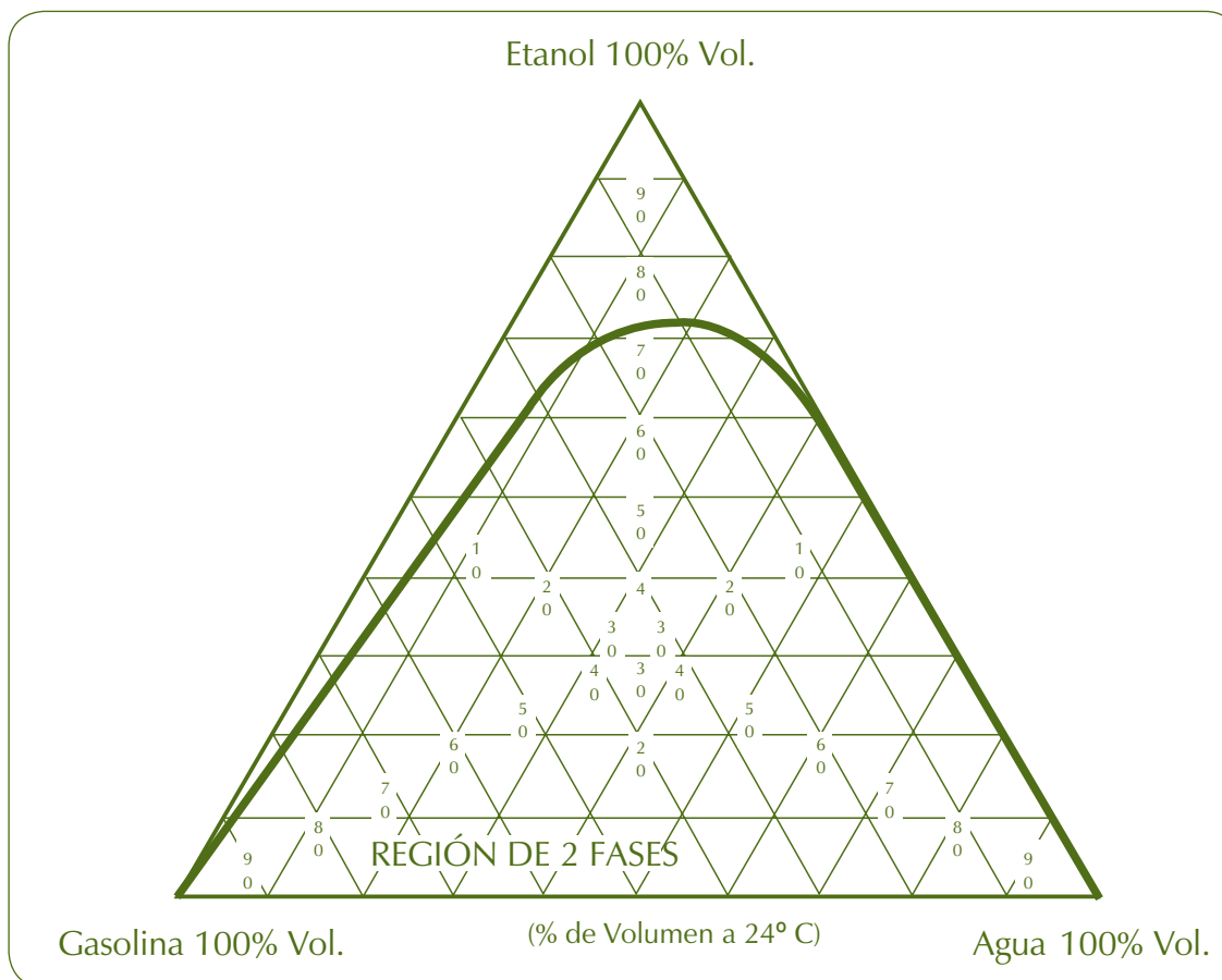
Figura 4 – Solubilidad de agua en mezclas gasolina/etanol
