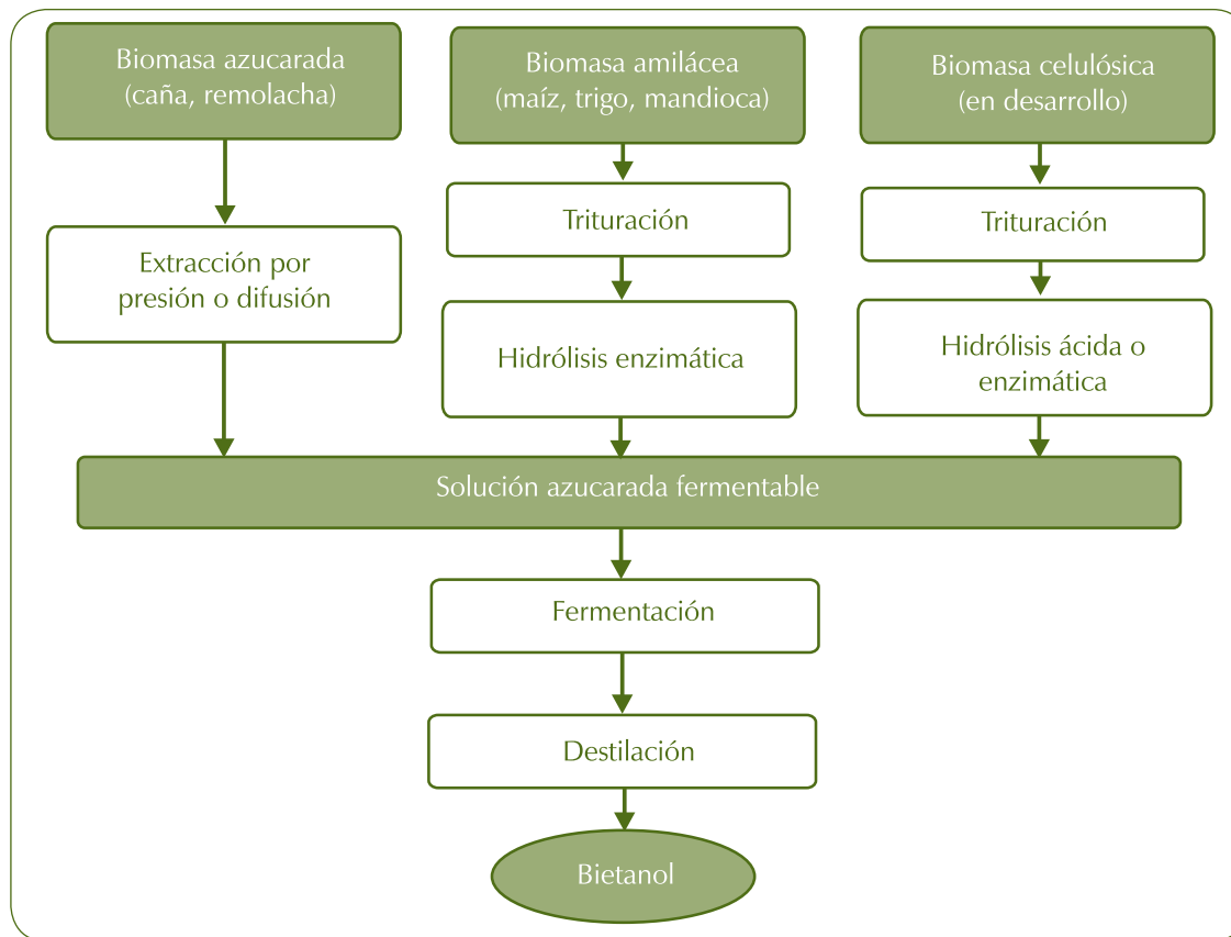
Figura 7 – Rutas tecnológicas para la producción de bioetanol
