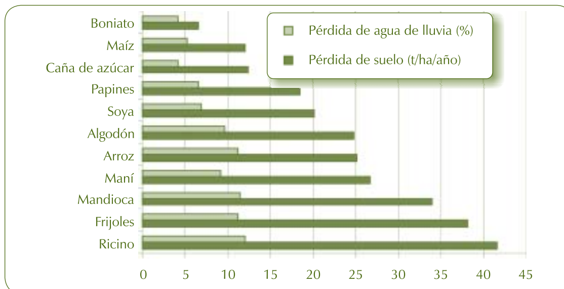
Gráfico 25 – Pérdidas de suelo y de agua de lluvia en algunos cultivos en Brasil
