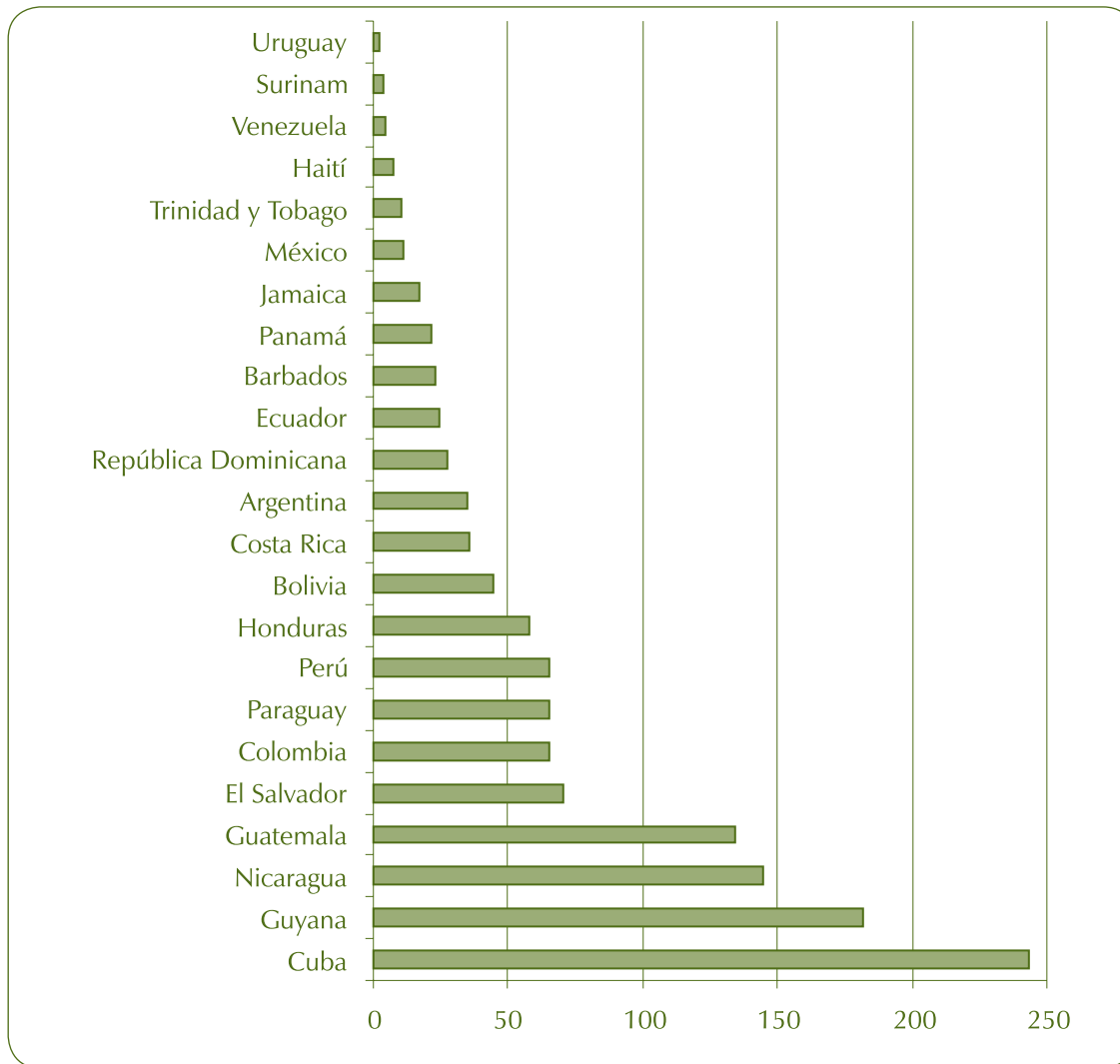
Gráfico 38 – Fracción de la demanda de bioetanol para agregar el 10% a la gasolina que se puede producir mediante la conversión de melaza disponible en la fabricación de azúcar
