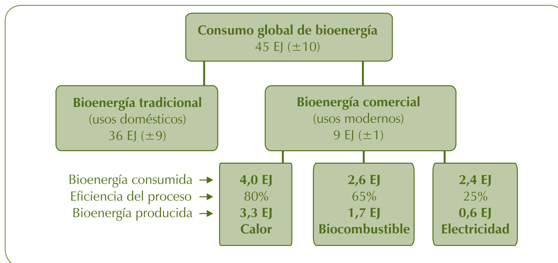
Figura 31 – Contribución de la bioenergía a la oferta primaria y secundaria de energía en el año 2007
