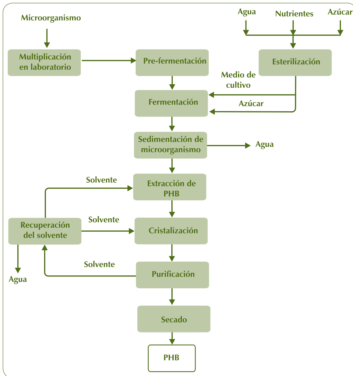
Figura 22 – Diagrama de flujo de la producción de PHB a base de azúcar de caña
