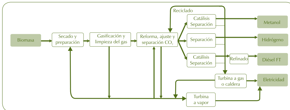
Figura 21 – Flujograma general para la producción de metanol, hidrógeno y diésel vía gasificación de biomasa (Fischer-Tropsch)
