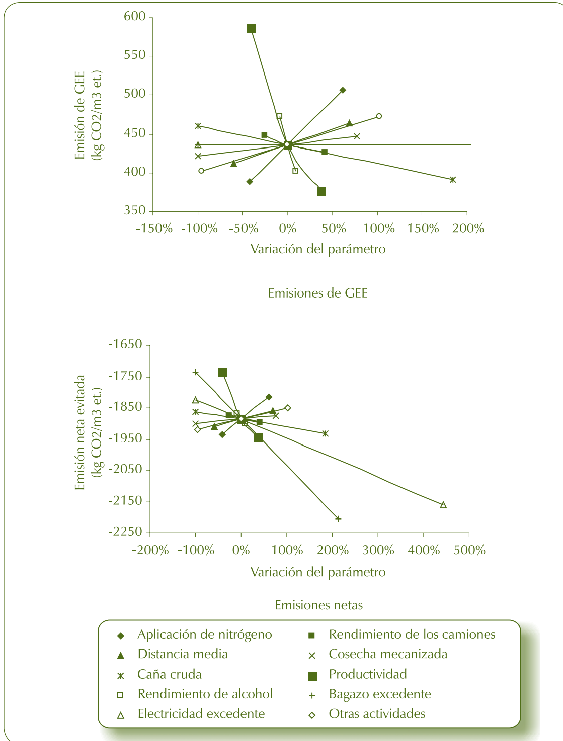
Figura 17 – Análisis de sensibilidad de las emisiones de GEE en la producción de bioetanol de caña de azúcar en el escenario actual (2005/2006)
