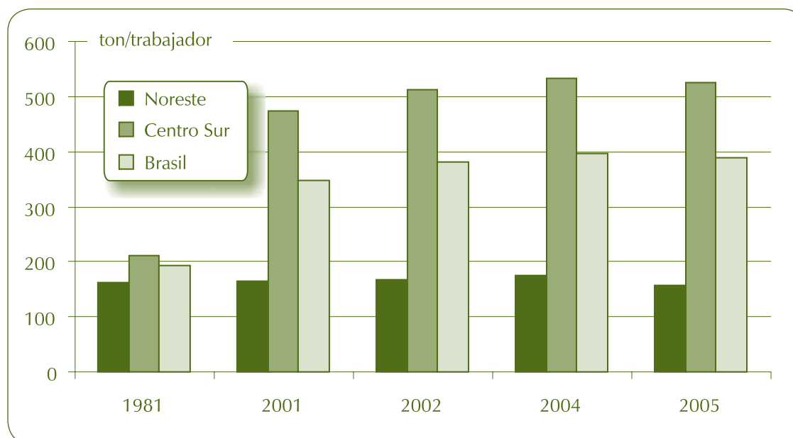
Gráfico 35 – Productividad promedio de los trabajadores de la agroindustria de caña en Brasil
