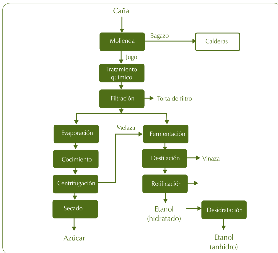
Figura 10 – Diagrama del movimiento de la producción de azúcar y bioetanol de caña
