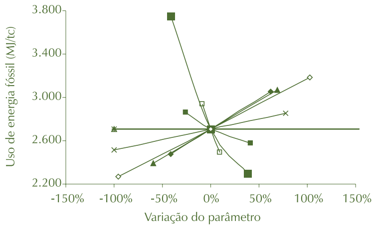
Figura 16 – Análise de sensibilidade para o uso e a relação de energia para o bioetanol de cana-de-açúcar no cenário atual (2005/2006)
