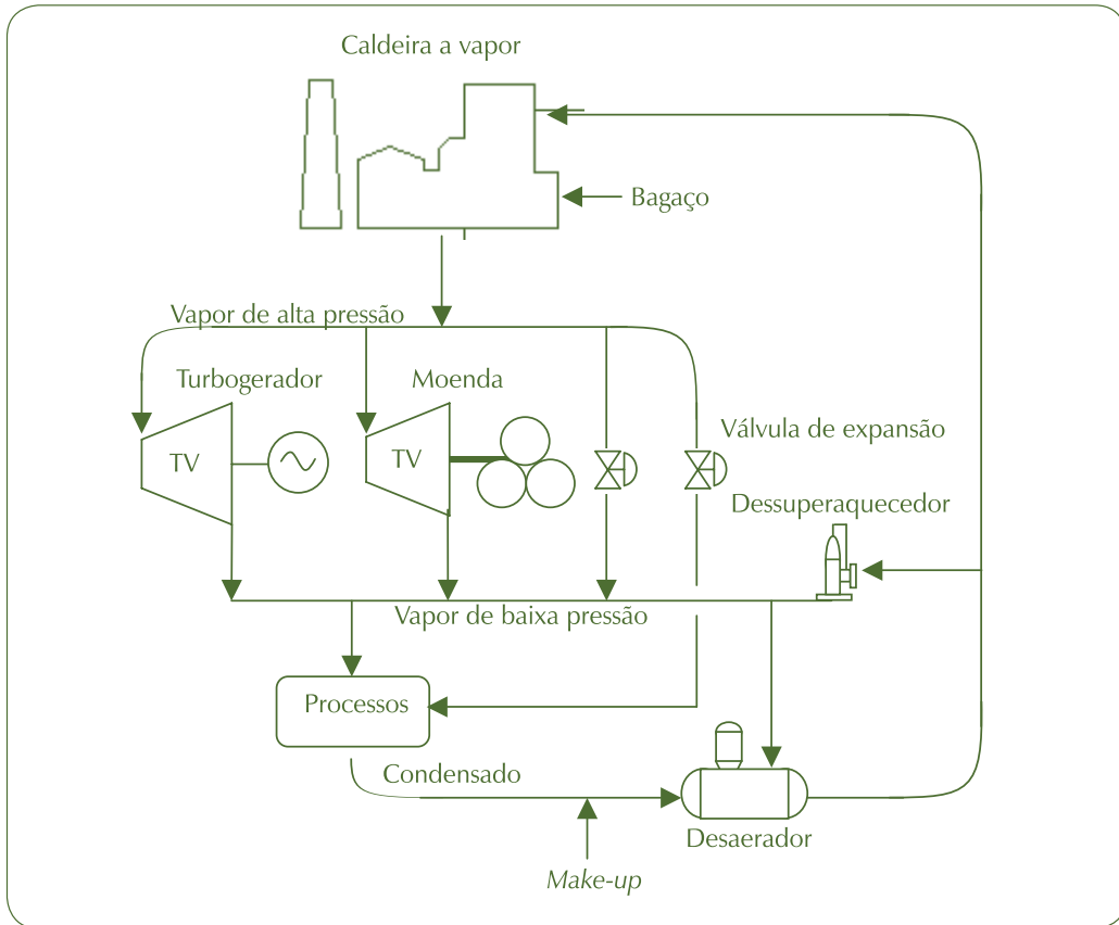
Figura 18 – Configuração usual do sistema de co-geração na agroindústria canvieira
