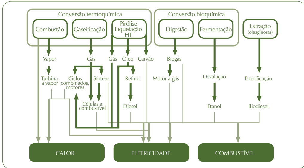
Figura 3 – Rotas tecnológicas para produção de bioenergia
