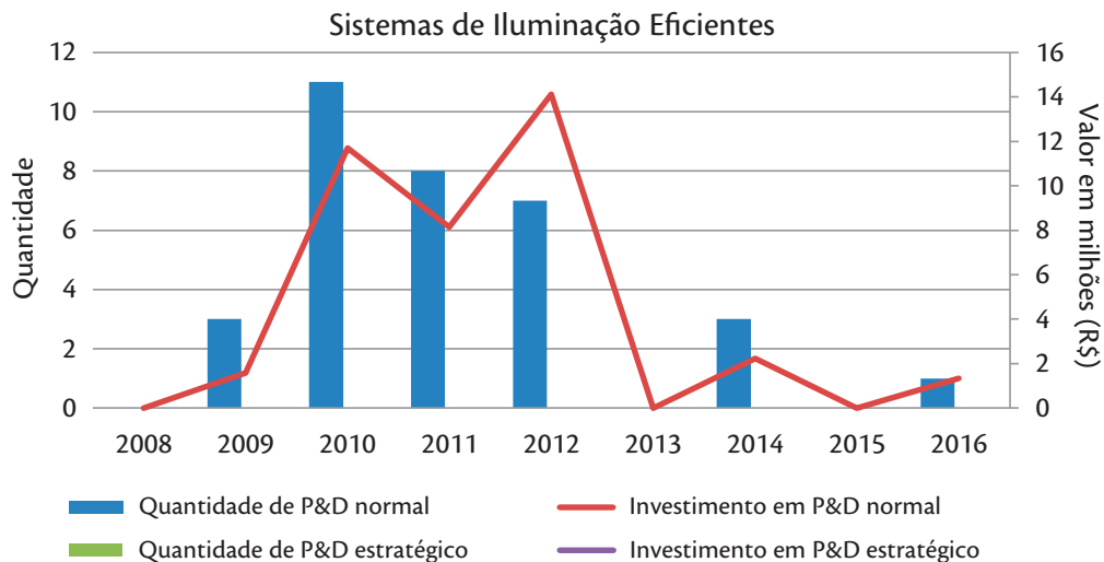
Gráfico 171 -Evolução da quantidade de projetos e valores investidos no P&D Aneel para a macrotemática Sistemas de Iluminação Eficientes no período de 2008 a 2016
