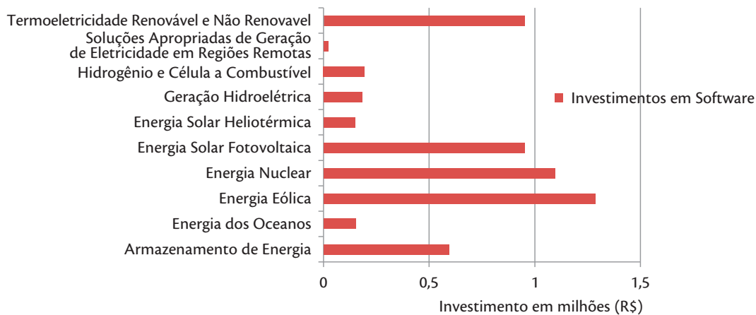
Gráfico 42 - Investimentos financeiros em softwares realizados nos laboratórios disponíveis às macrotemáticas do GT Geração de Energia Elétrica e Armazenamento de Energia, no período de 2014 a 2016
